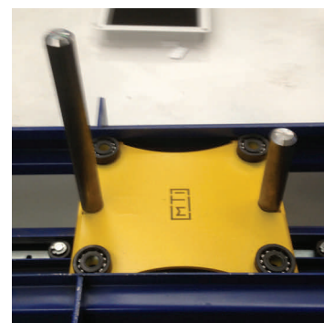
Instalación de transportador SLF 50 +150/300 en la empresa Faurecia (Barcelona)
